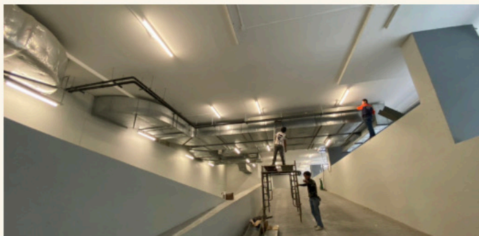
งาน ติด S-OASIS ร้าน MOM'S TOUCH ระบบ VRF ยี่ห้อ LG จำนวน 1 SYSTEM 3 GCU 1CDU
